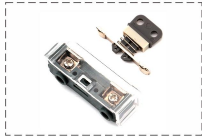
QKS9 Schindler door contact
