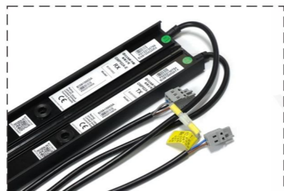
GMP02A-W Hitachi door sensor
