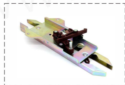
3300AP Fermator schindler door vane
