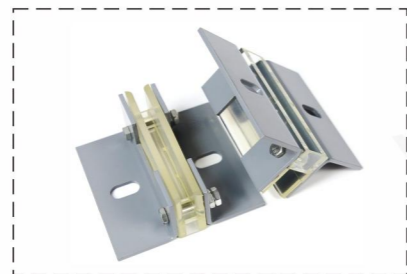
120*10/16 Otis guide shoe
