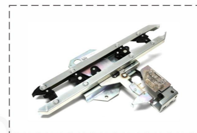
CDL-CARECC200 Fermator door vane
